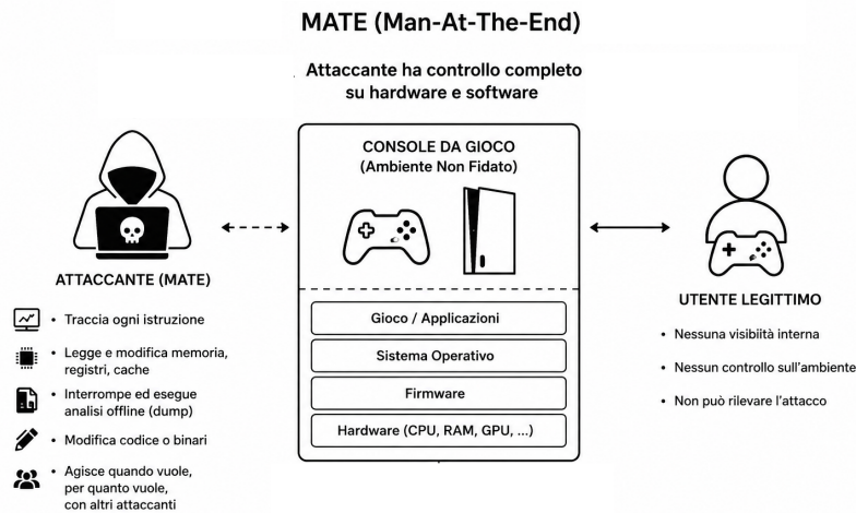
Figura 2: Schema concettuale attacco man-at-the-end
